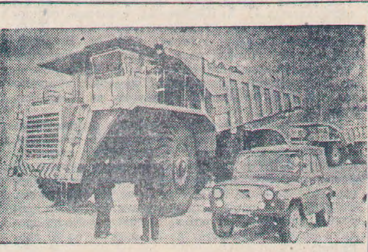
Мурманская область. В карьерах Ждановского рудника запольного горнометаллургического комбината «Печенганикель» успешно проходят испытания 110-тонного автосамосвала «БелАЗ» (на снимке). Длина машины свыше 11 метров, ширина более 6 метров, мощность двигателя — 1300 лошадиных сил. Автосамосвал способен перевезти за год миллион тонн горной породы и заменить в карьере 3—4 автомобиля «БелАЗ-548».
